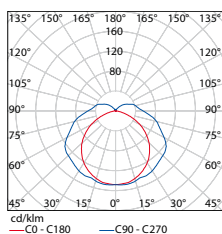
MIRA 2x18W
