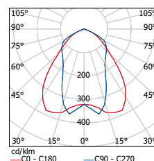
MH5 E40
