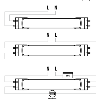
Schématu možného zapojení:
