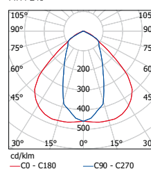
MH4 E40
